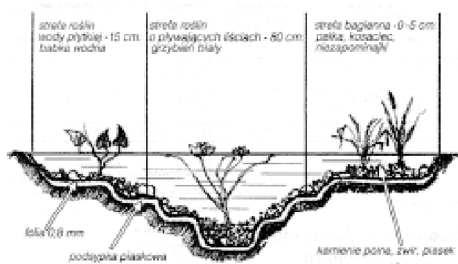
Przekrój stawki
